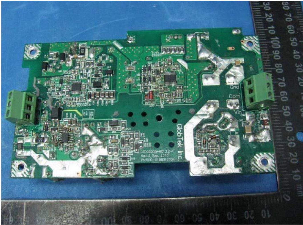
内部照片
