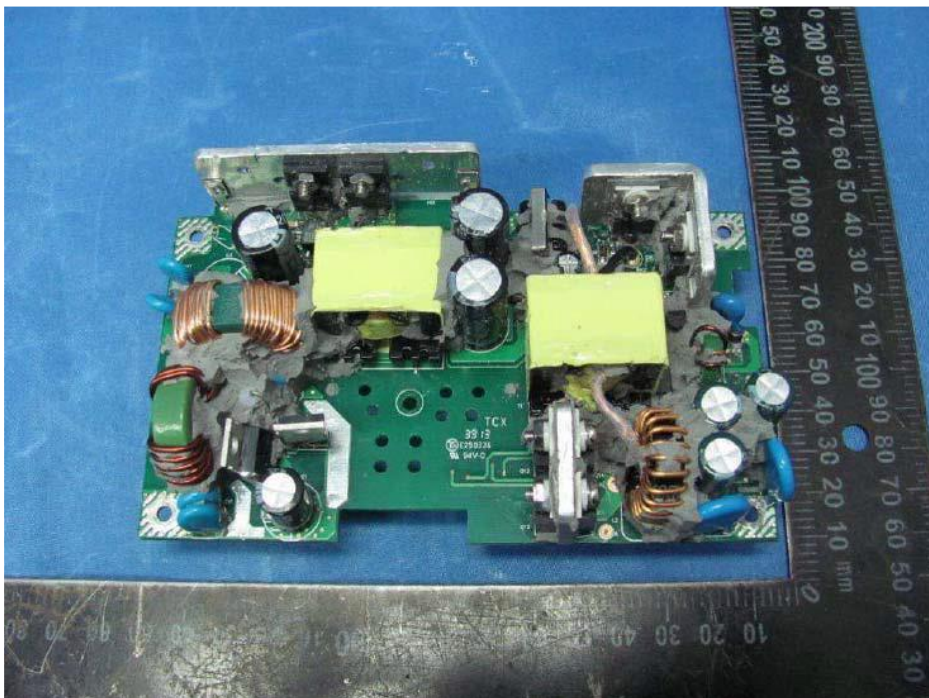
内部结构
