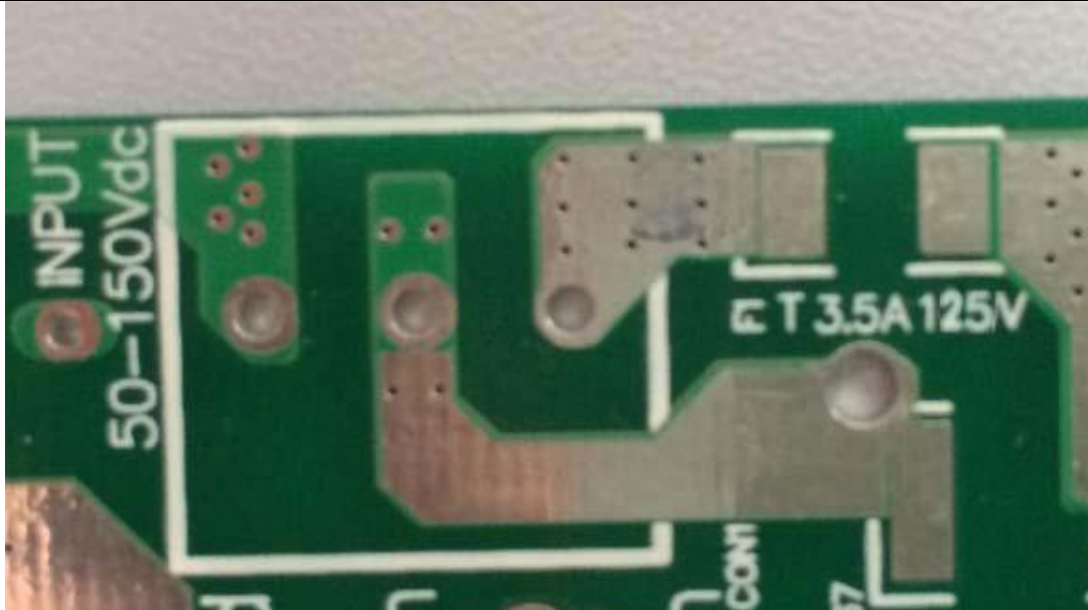
熔断器标识
