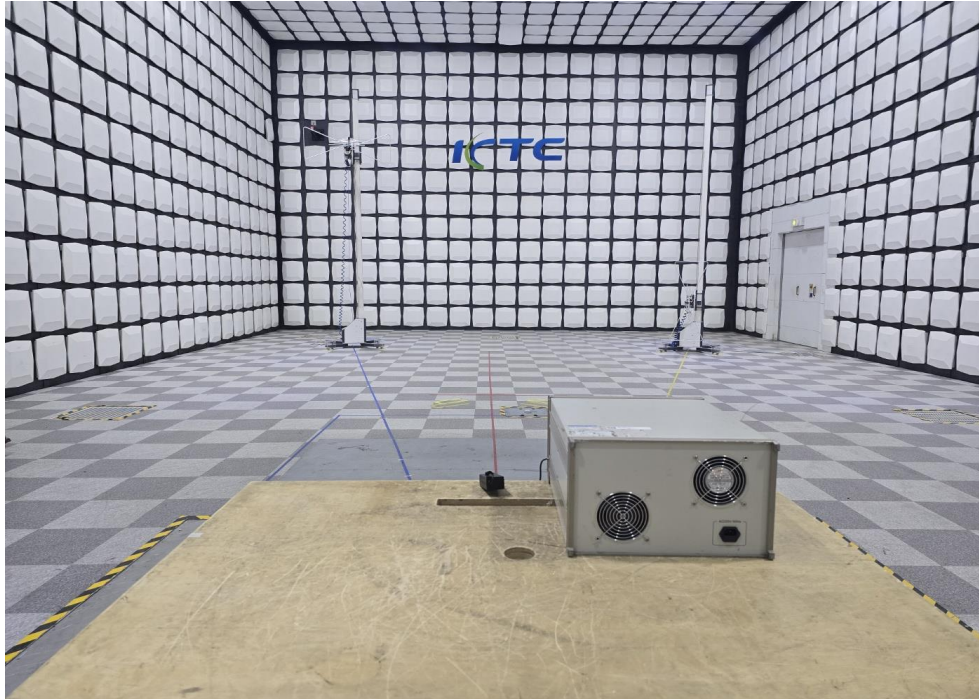
<복사성 방출-전면>
