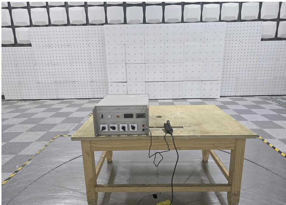
<복사성 방출-후면>
