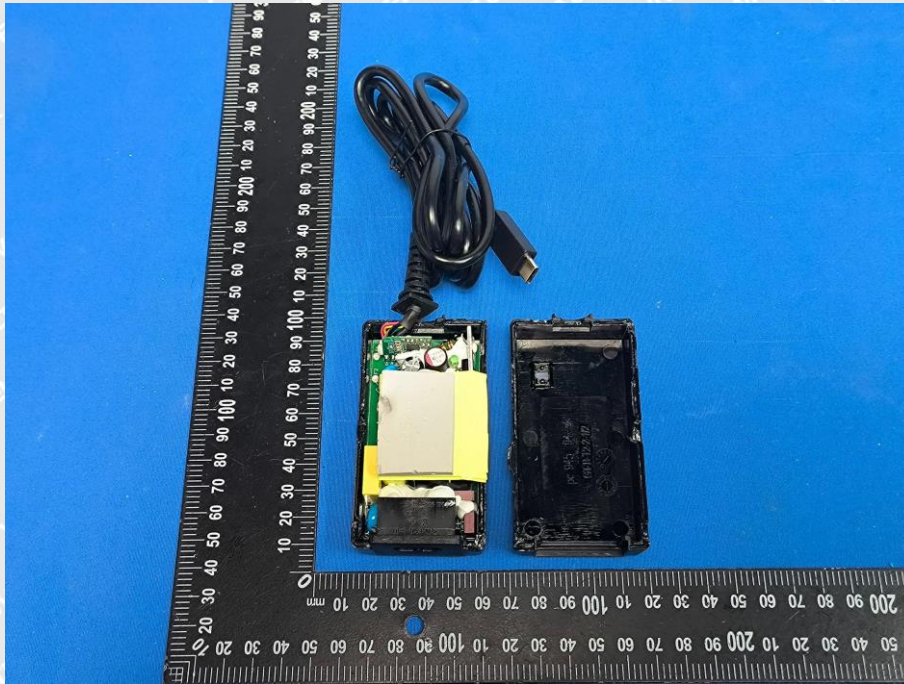
GTM96181-36PD-PPS-T2
