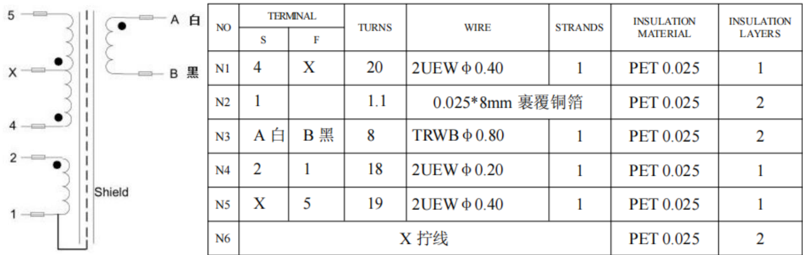
变压器内部结构图（型号：TF102）：
