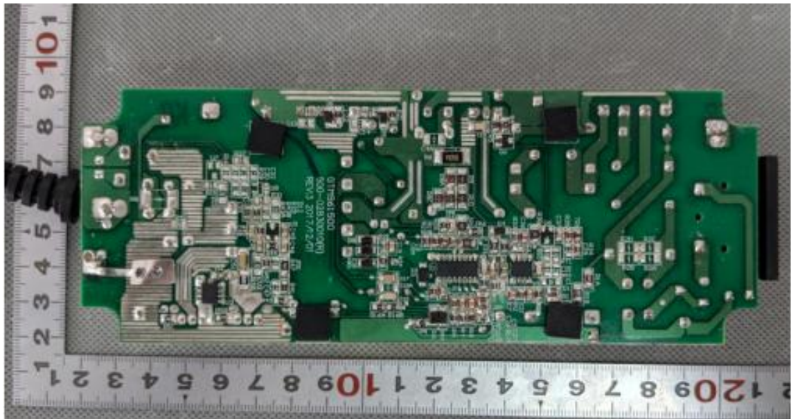
电源板（GTM961600P16012-T3A）
