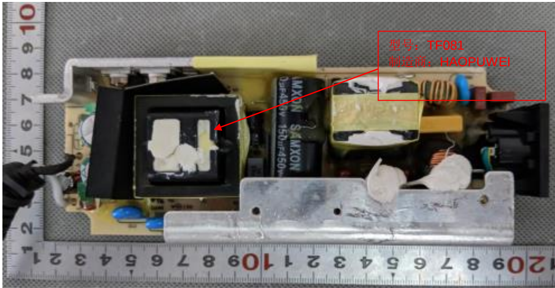
电源板（GTM961600P16012-T3A）
