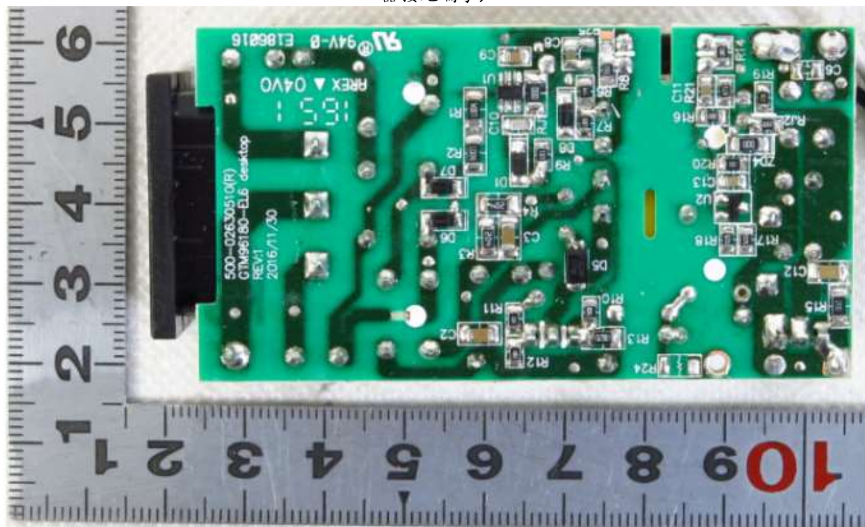
内部结构 (背面)
