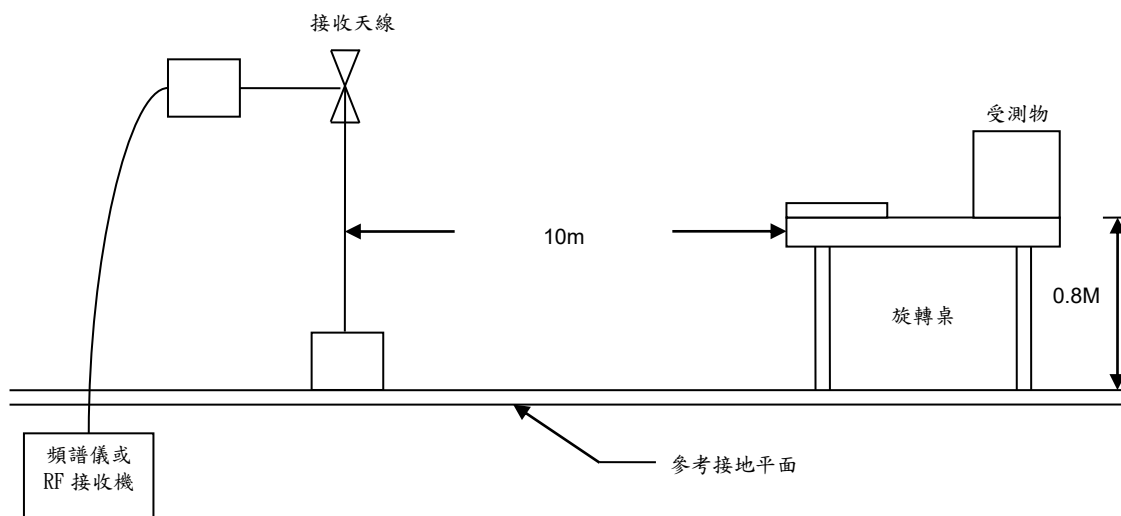
1GHz 以下測試擺設圖
