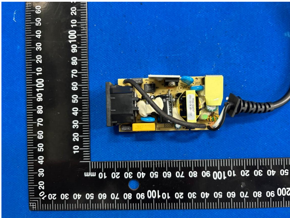
電路板零件面一(型號 GTM96180-1817.9-5.9-T3)
