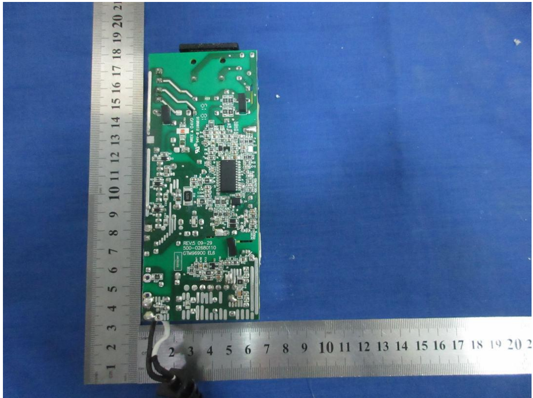
電路板零件面 (情況2之功能性接地型照片)
