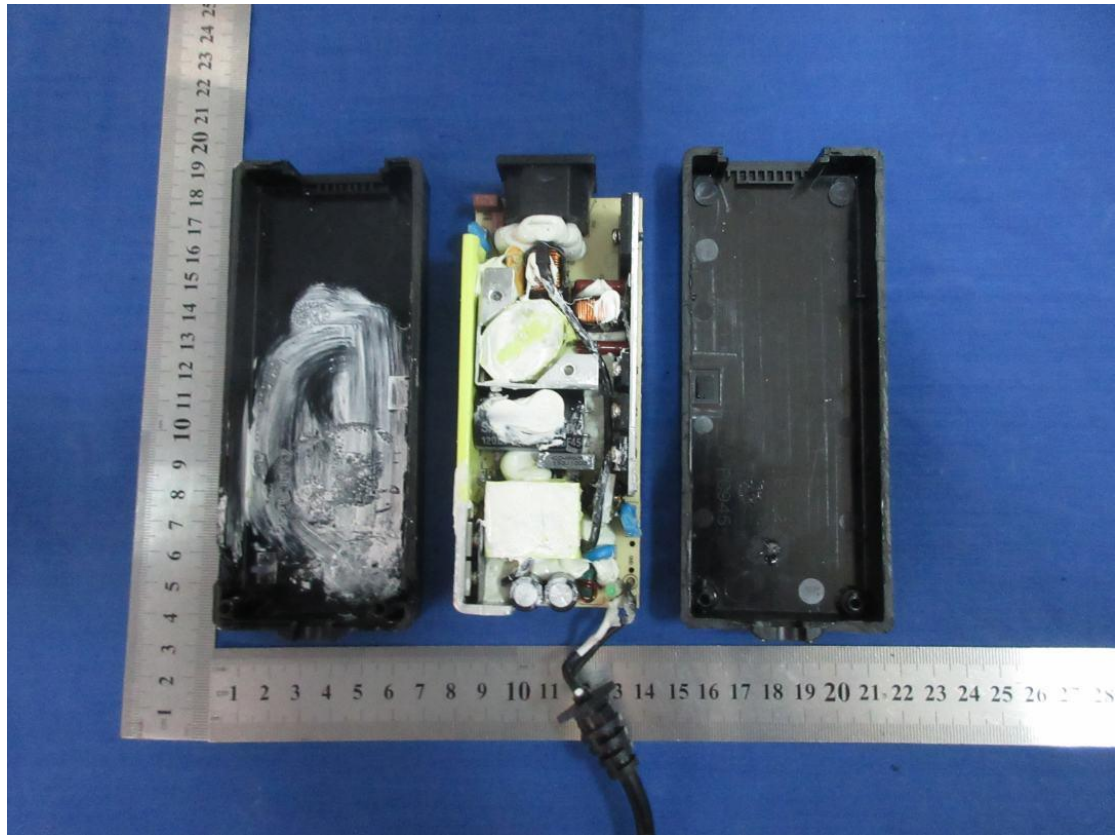
內部正視圖二
