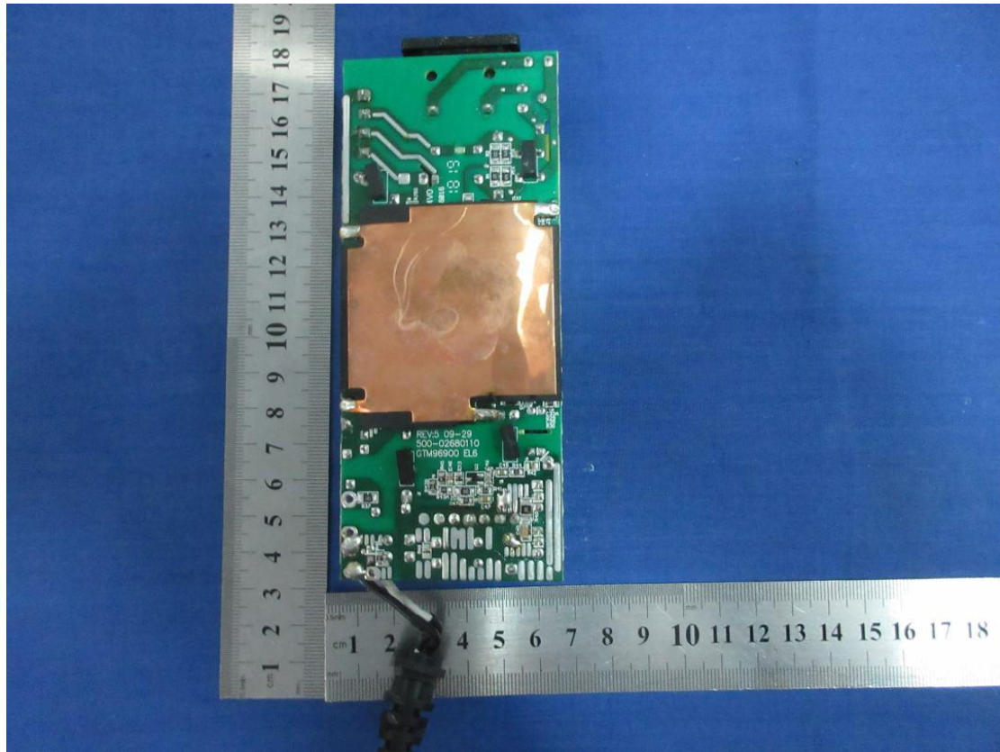
電路板零件面 (情況1之功能性接地型照片)
