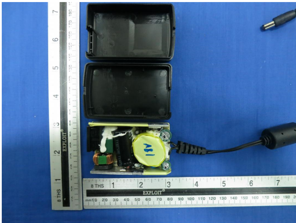
內部正視圖二
