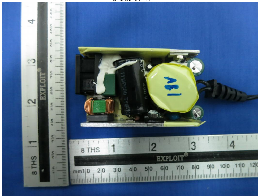
電路板元件面
