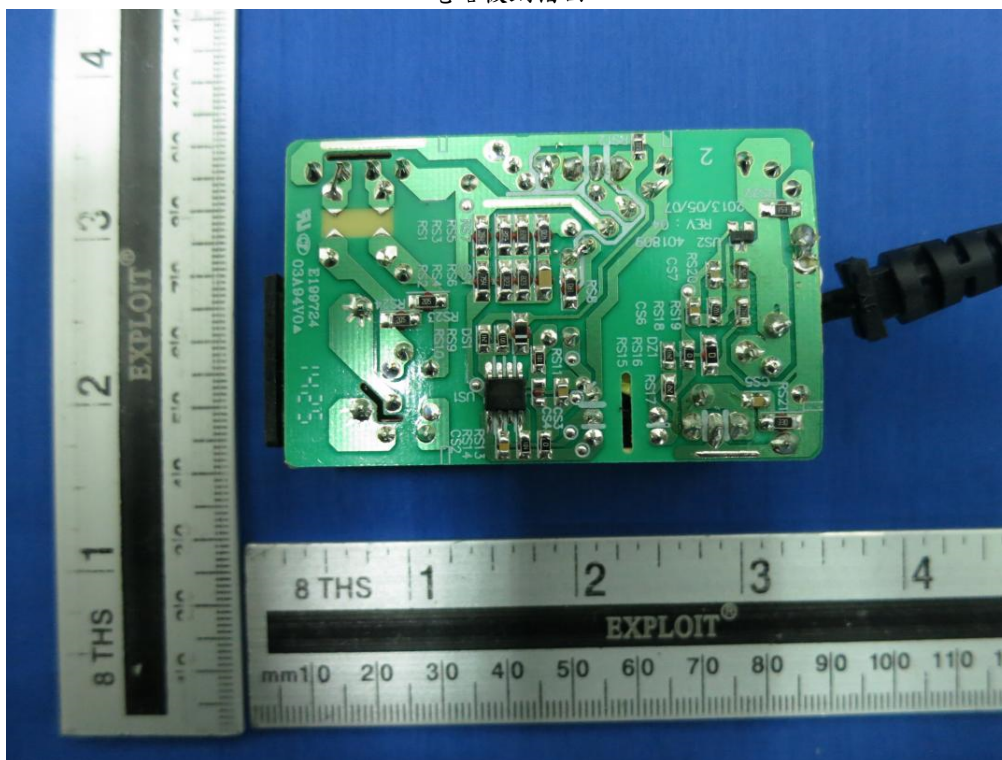
電路板銅箔面
